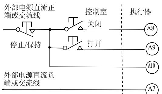
图 4-6 保持式打开、关闭、停止控制
