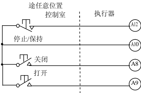
图 4-3 保持式打开、关闭、停止控制
