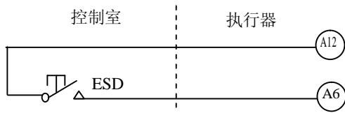
图 4-11 单线 ESD 控制，高电平有效。
