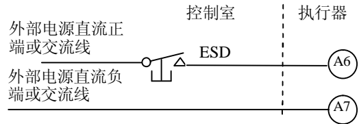
图 4-14 双线 ESD 控制，低电平有效。
