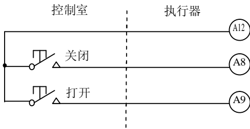
图 4-1 点动式打开/关闭控制，执行器可以停在中途任意位置
