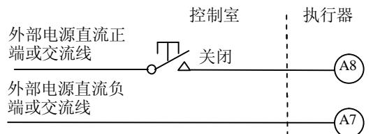
图 4-10 双线控制，有信号关，无信号开。
