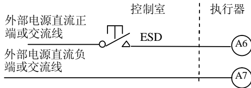
图 4-13 双线 ESD 控制，高电平有效。
