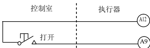
图 4-7 双线控制，有信号开，无信号关。
