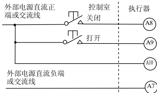
图 4-5 保持式打开 / 关闭控制，行程可逆，但不能停在中途位置
